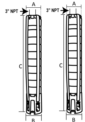
Acoplamiento NEMA 6" Fig. 1
